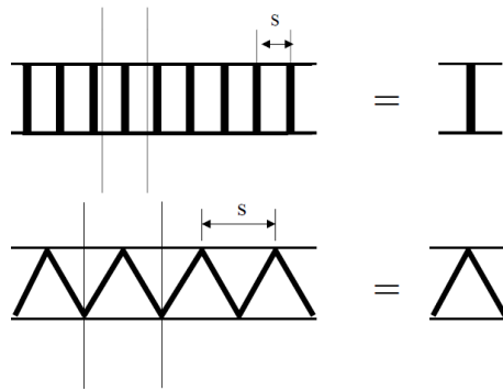
圖 III 2-12 擠壓板
