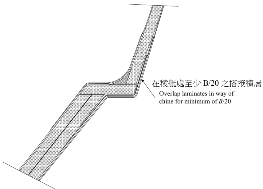
圖 III 2-37 階梯式稜艫-補土半徑
