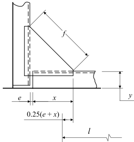
圖 III 1-5 腋板
