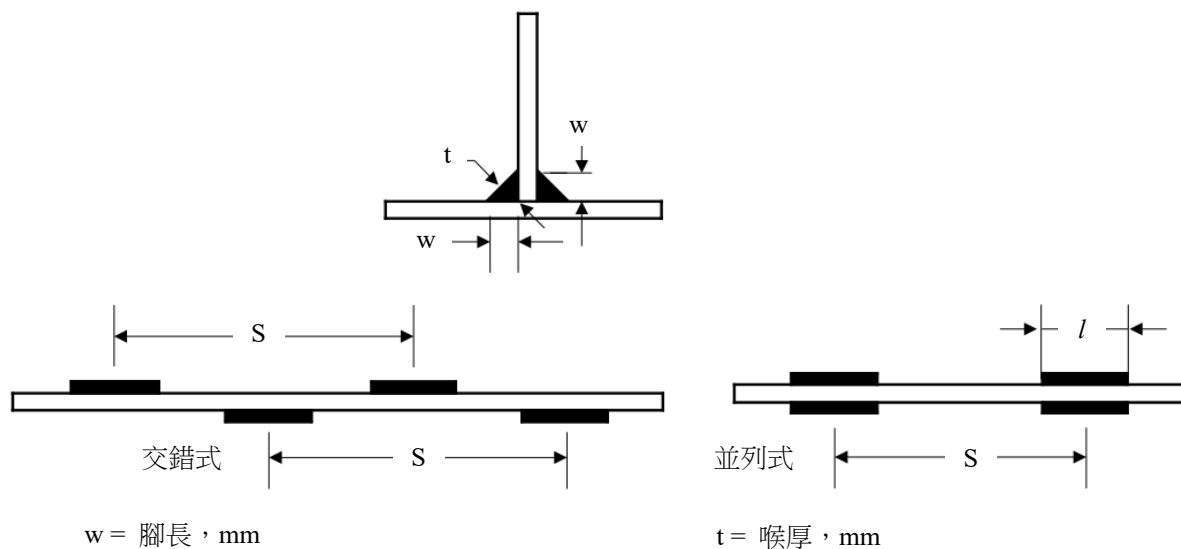
圖 II 2-5 斷續填角銲
