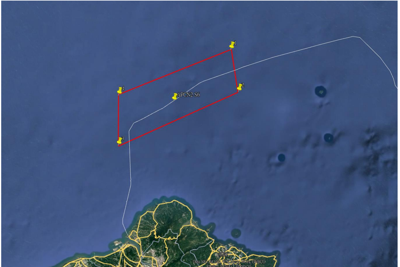
圖二：APCN2 S6 海纜故障修理工作範圍
