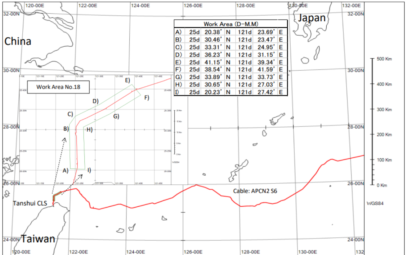
圖二(B)：APCN2 S6-18 海纜故障修理工作範圍 (座標系統 WGS84)
