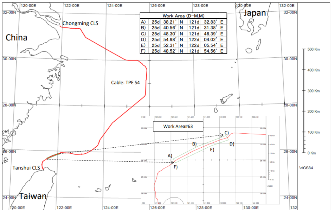
圖二(A)：TPE S4-63 海纜故障修理工作範圍
