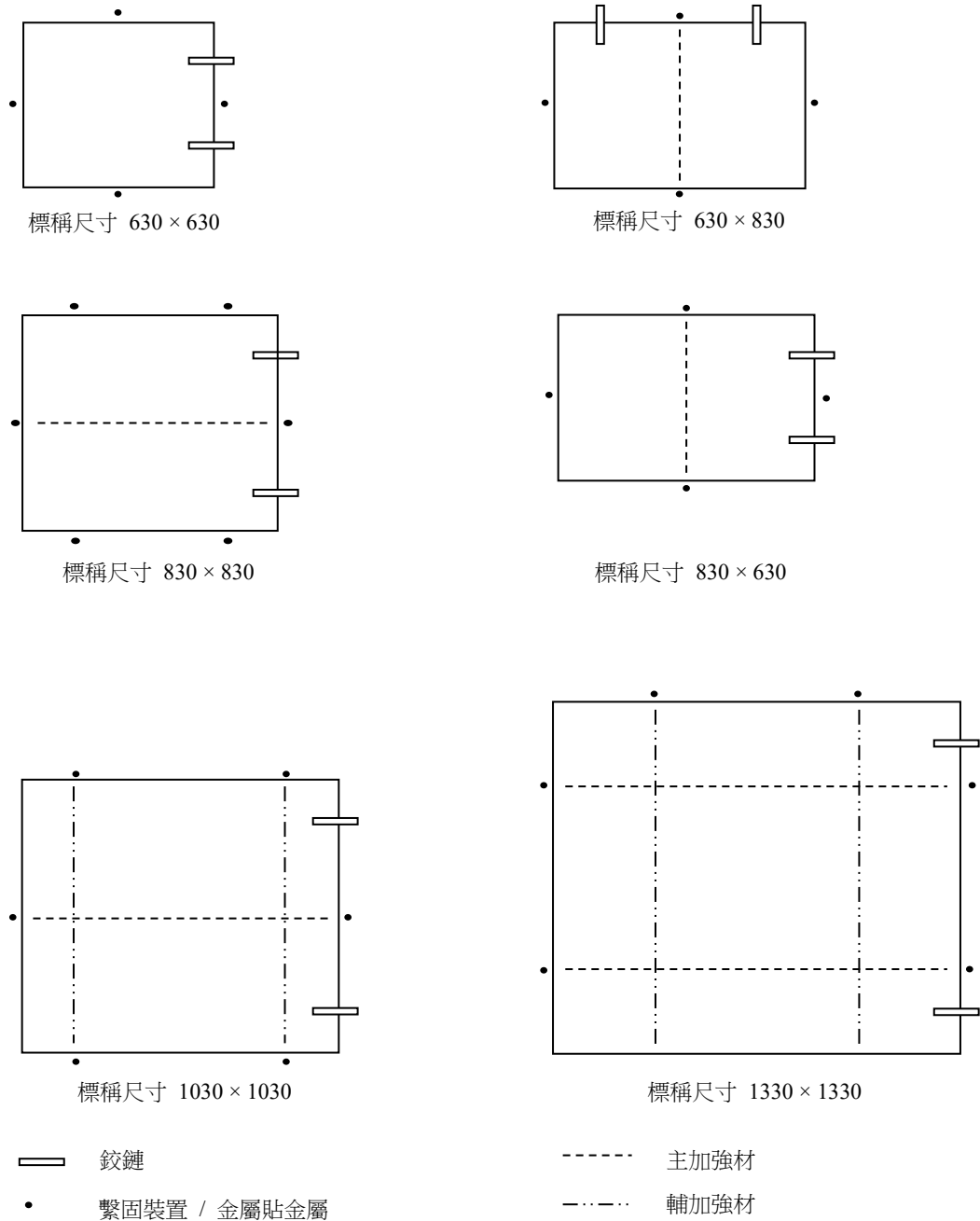
圖 II 27-1 加強材之布置
