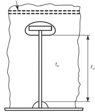
(b) 切形槽連接
