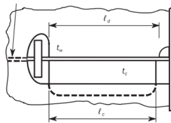
(e) 補板和直接連接
