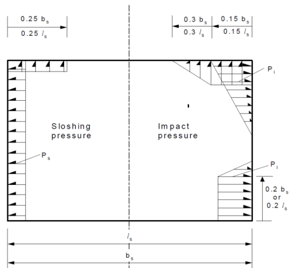
圖 II 33-3 壓力分佈
