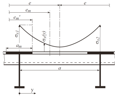
圖 II 17-5 垂直主支撐構件腹板之加強
