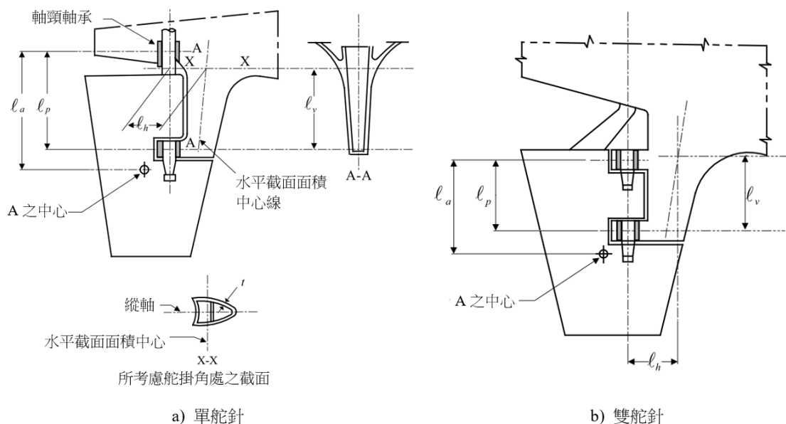
圖 III 2-44 舵掛角
