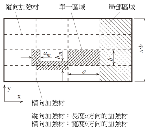
圖 II 17-3 嵌板的一般布置
