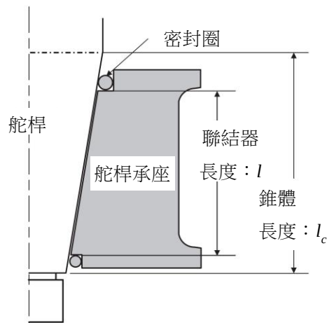
圖 II 24-7C 錐體長度及聯結器長度
