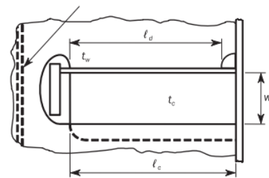
(d) 補板的直接連接
