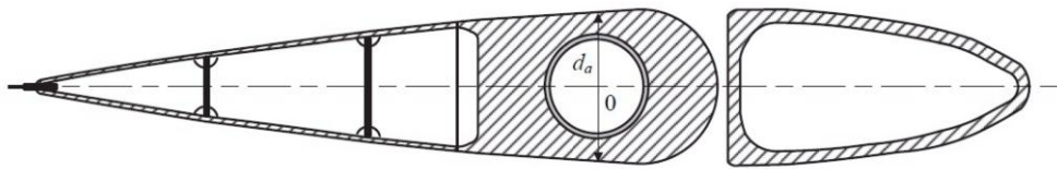
圖 II 24-7B 舵桿承座之外徑( d_a )量測
