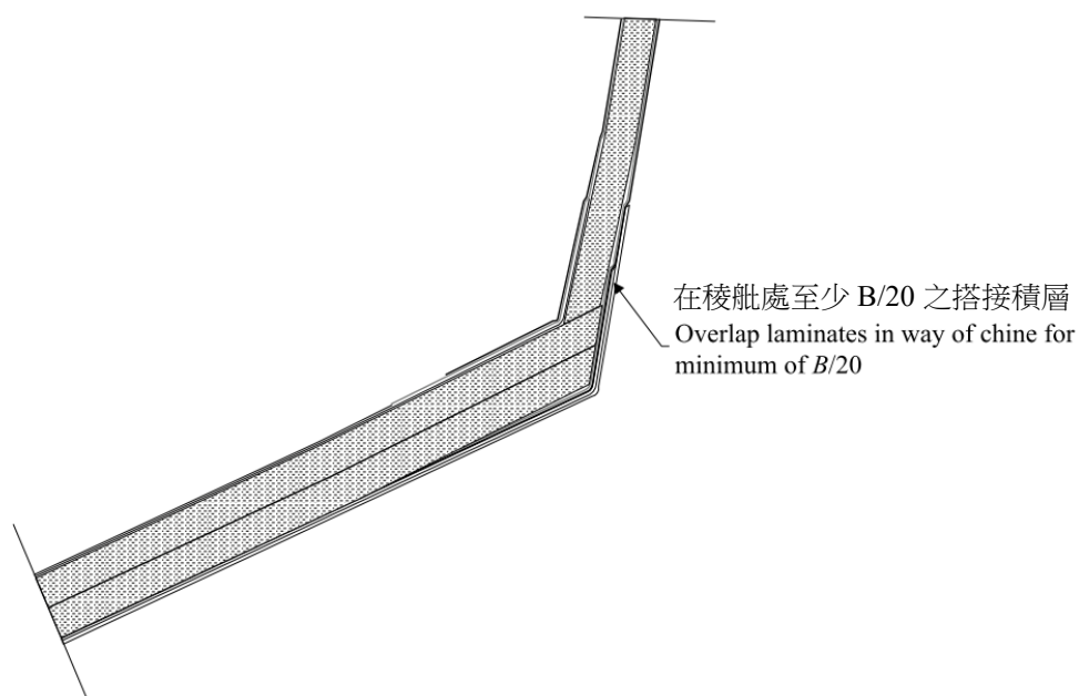
圖 III 2-35 稜艭或艭橫板-三明治構造
