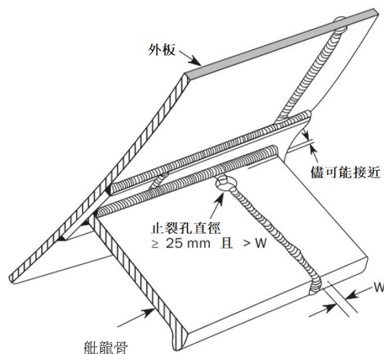
圖 II 1-8 舢龍骨構造
