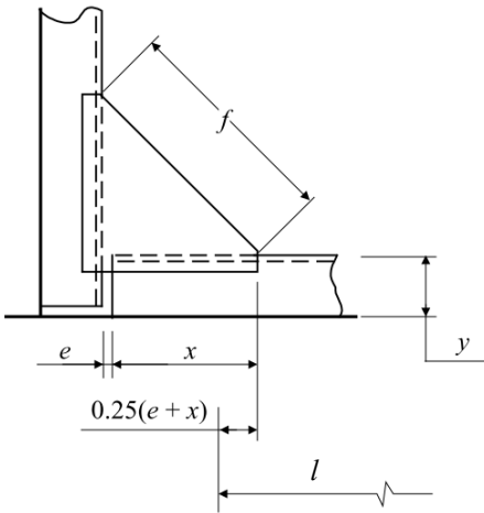
圖 III 1-5 腋板
