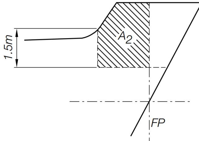
圖 II 25-3 屏幕、舷牆等之有效面積
