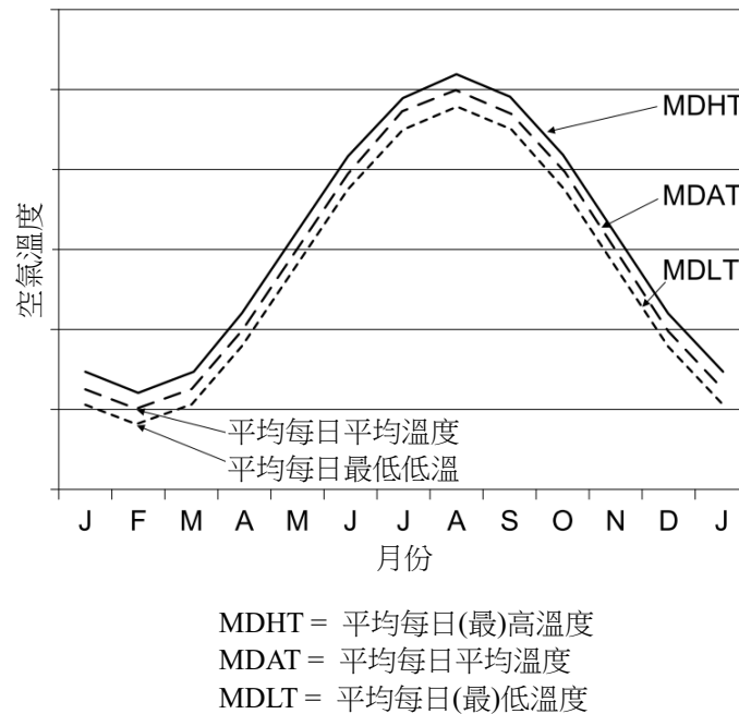
圖 III 1-1 溫度通用定義
