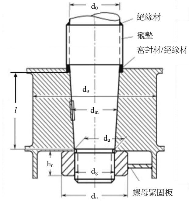
圖 II 24-7A 有鍵錐形聯結器
