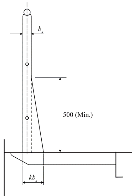
圖 III 2-56 欄杆支柱
