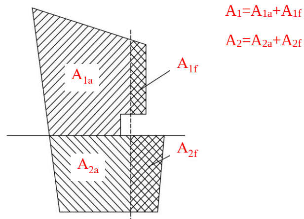
圖 II 24-4 缺角舵葉
