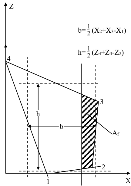
圖 II 24-3 完整舵葉
