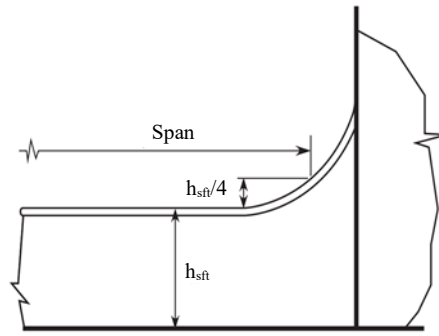
圖 II 1-4 沿著肋板邊緣具有連續面板之局部支撐構件的有效彎曲跨距
