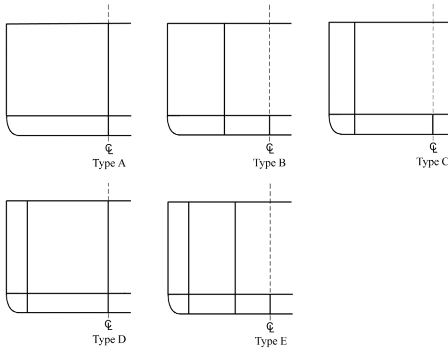
圖 II 3-6 有縱向隔艙壁之船舶的類型
