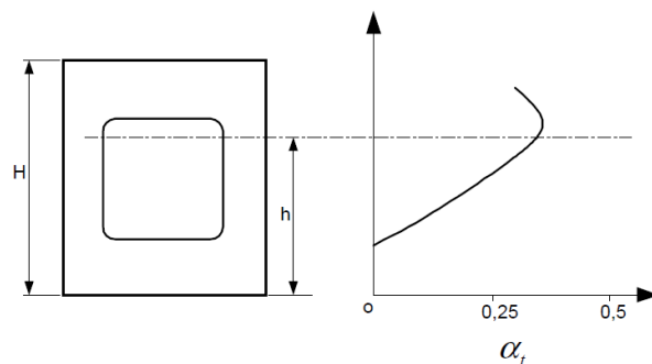
圖 II 33-1 制水艙壁係數
