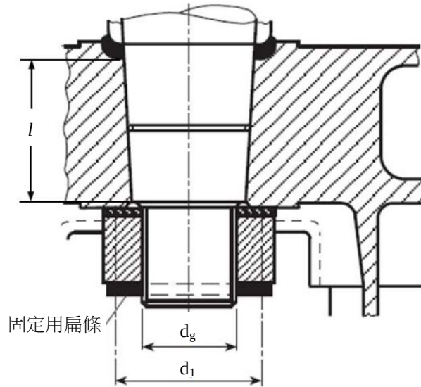
圖 II 24-8 無鍵錐形聯結器
