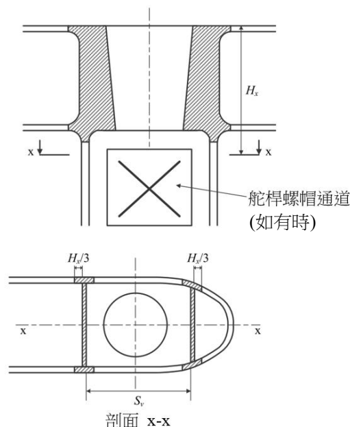
圖 III 2-49 舵葉與舵桿承座連接處剖面
