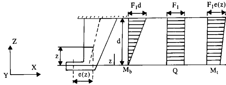
圖 II 2-3 舵掛角負荷
