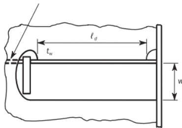
(c) 沒有補板的直接連接
