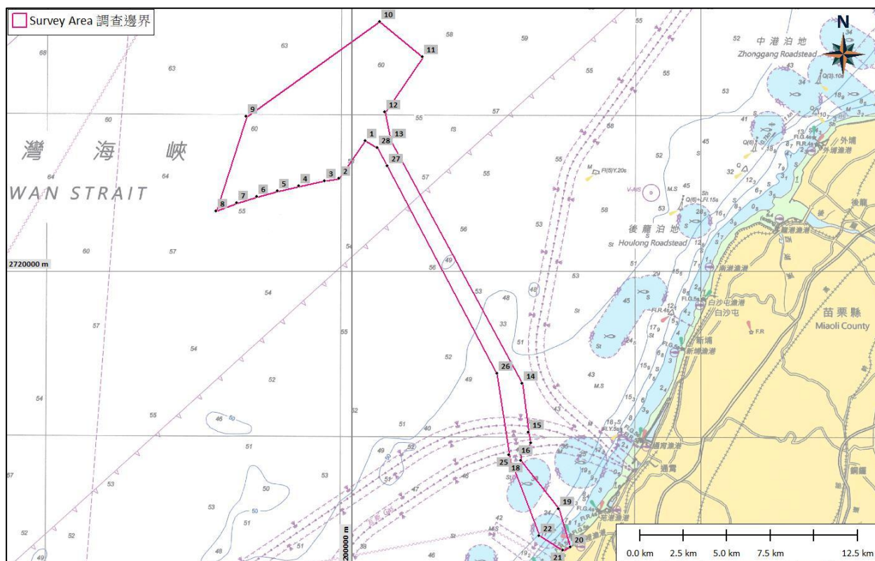
圖 1 作業區域位置圖(Figure 1-Layout of Work Area)
